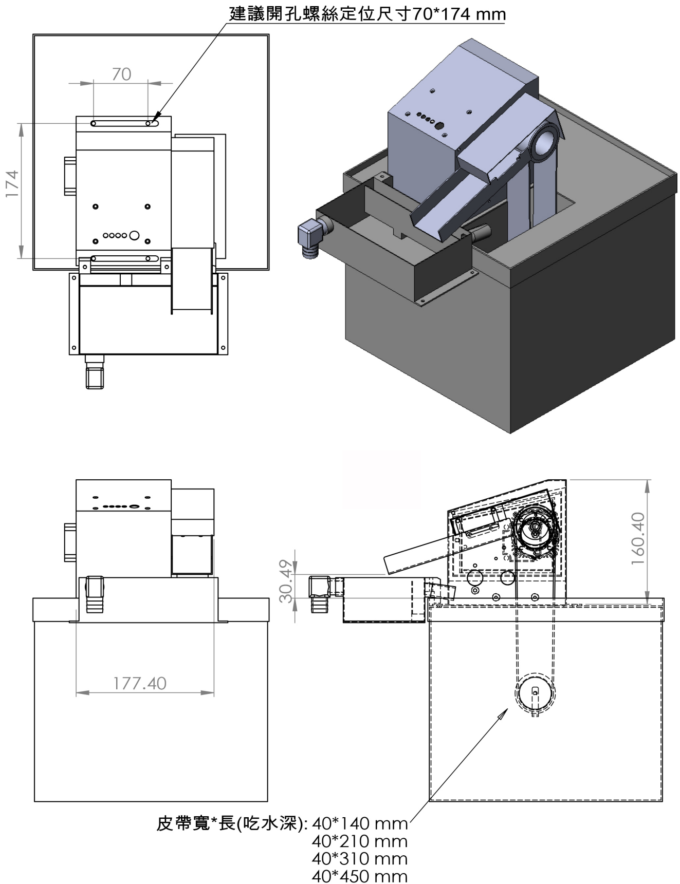
皮帶式安裝示意圖
